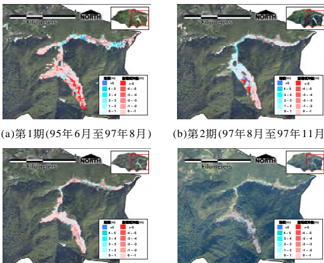
(a) 第1期(95年6月至97年8月) (b) 第2期(97年8月至97年11月) (c) 第3期(97年11月至98年10月) (d) 第4期(98年10月至99年11月) 圖十五 蘇樂集水區之土砂運移分析成果圖
